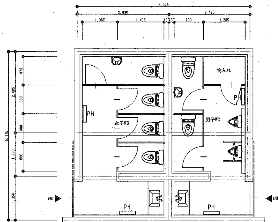
改修後平面図
